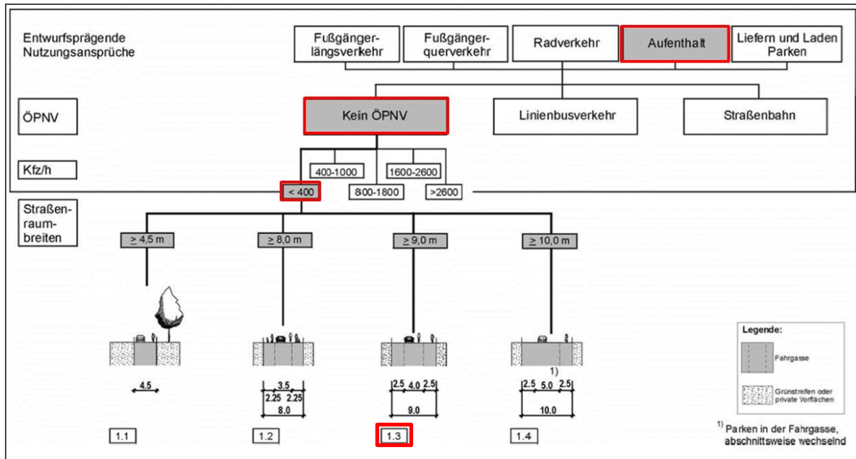
Abbildung 17: Mögliche Querschnitte für Wohnwege nach RAS t
